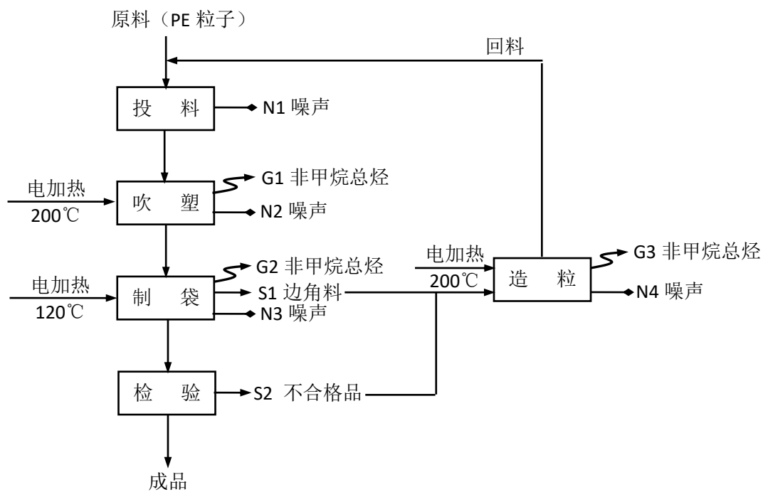
图 2-2 塑料包装袋生产工艺流程及产污环节图
