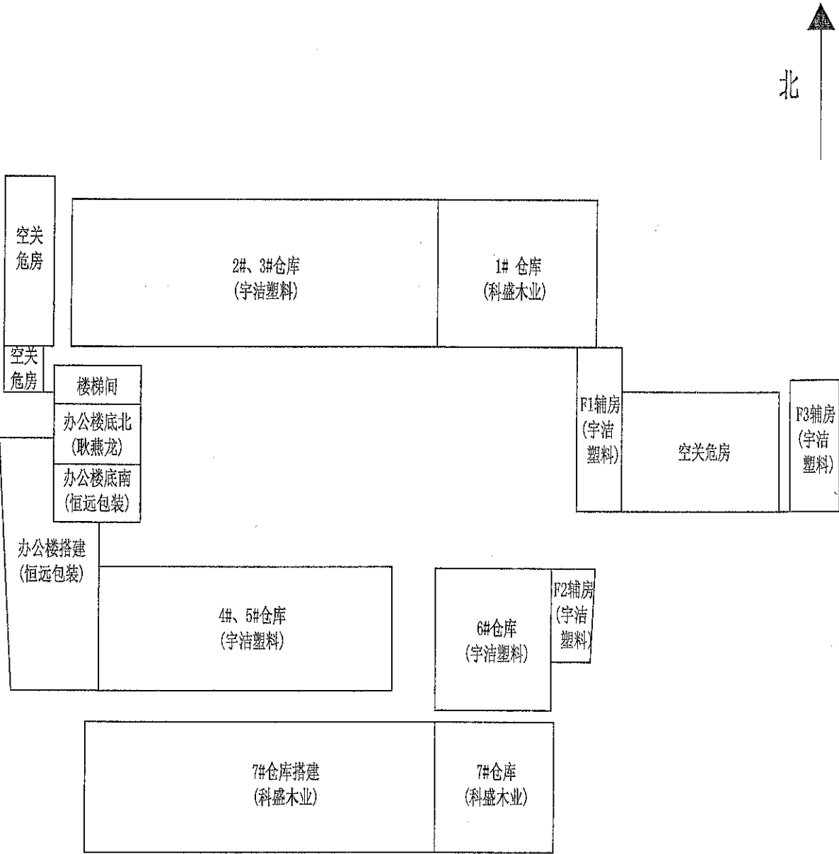
山观西街124号山观粮管所(中库)平面示意图
