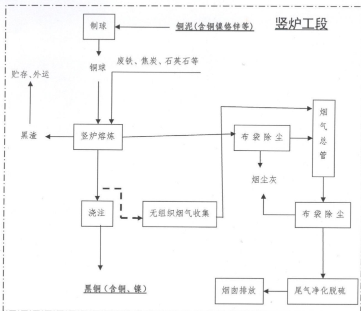
文字描述及工艺流程图
