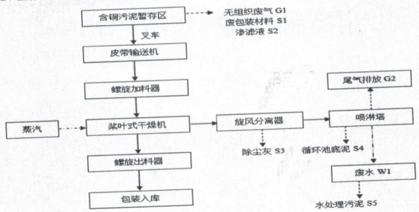
图 2 主体工程生产工艺流程图
